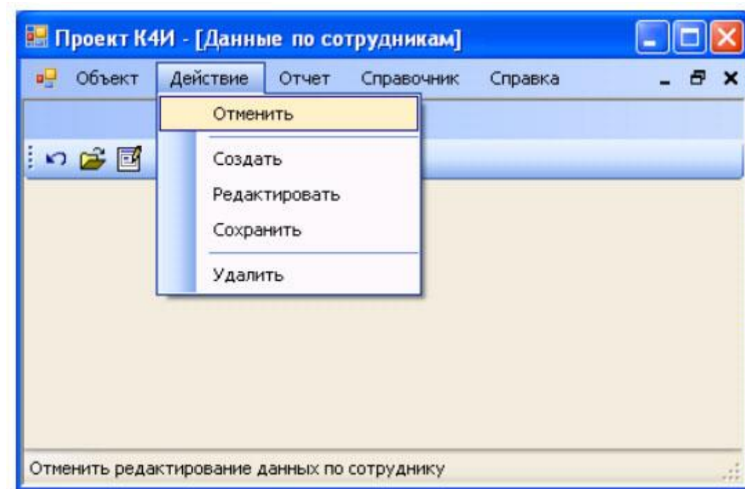
Рис. 6.6. Экранная форма со строкой состояния
