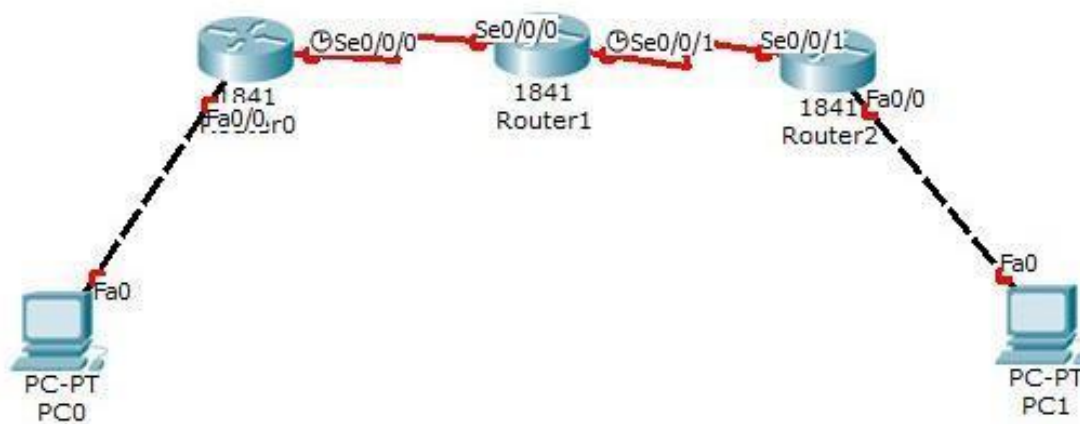
Рис. 4.1 – Топология сети
