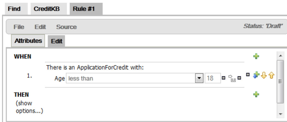
Рисунок 18 - Добавленное ограничение на поле Age
