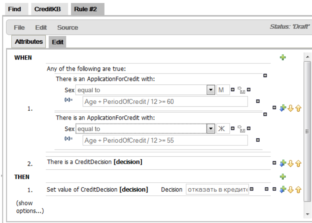
Рисунок 24 - Законченное правило Rule #2
