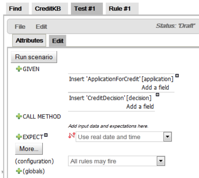
Рисунок 33 - Тест Test #1 и входные факты
