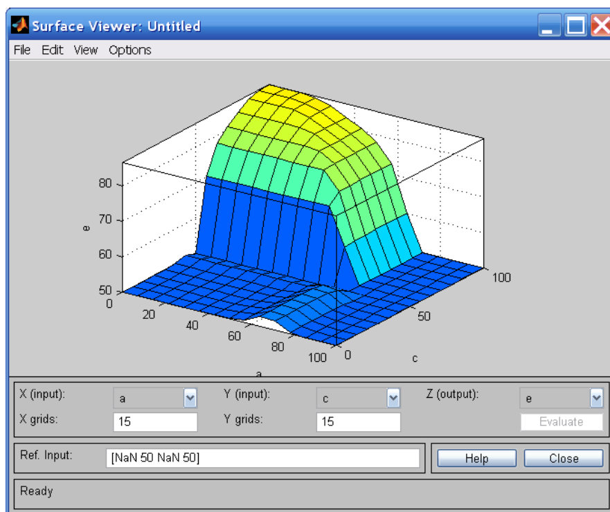
Рисунок 11 – Окно «Просмотр поверхности» с измерениями a, c, e и поверхностью отклика системы
