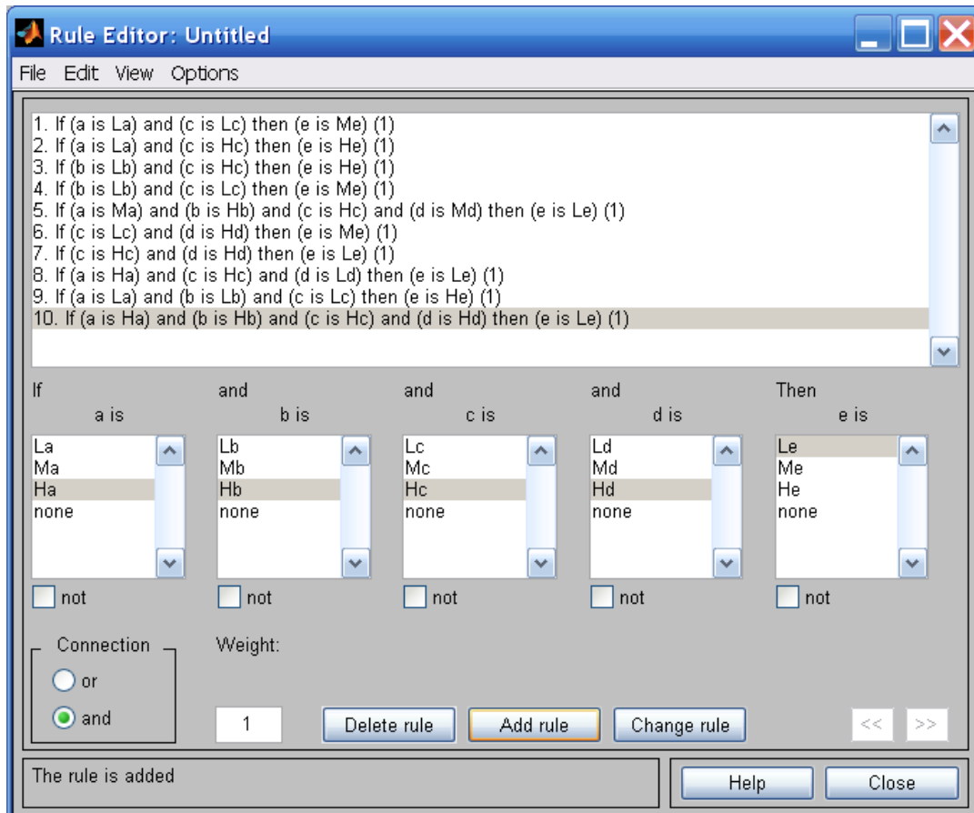
Рисунок 6 – Окно редактора правил
