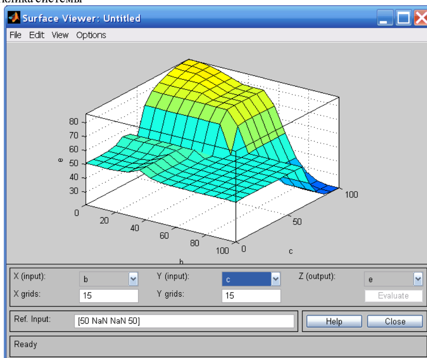
Рисунок 12 – Окно «Просмотр поверхности» с измерениями b, c, e и поверхностью отклика системы
