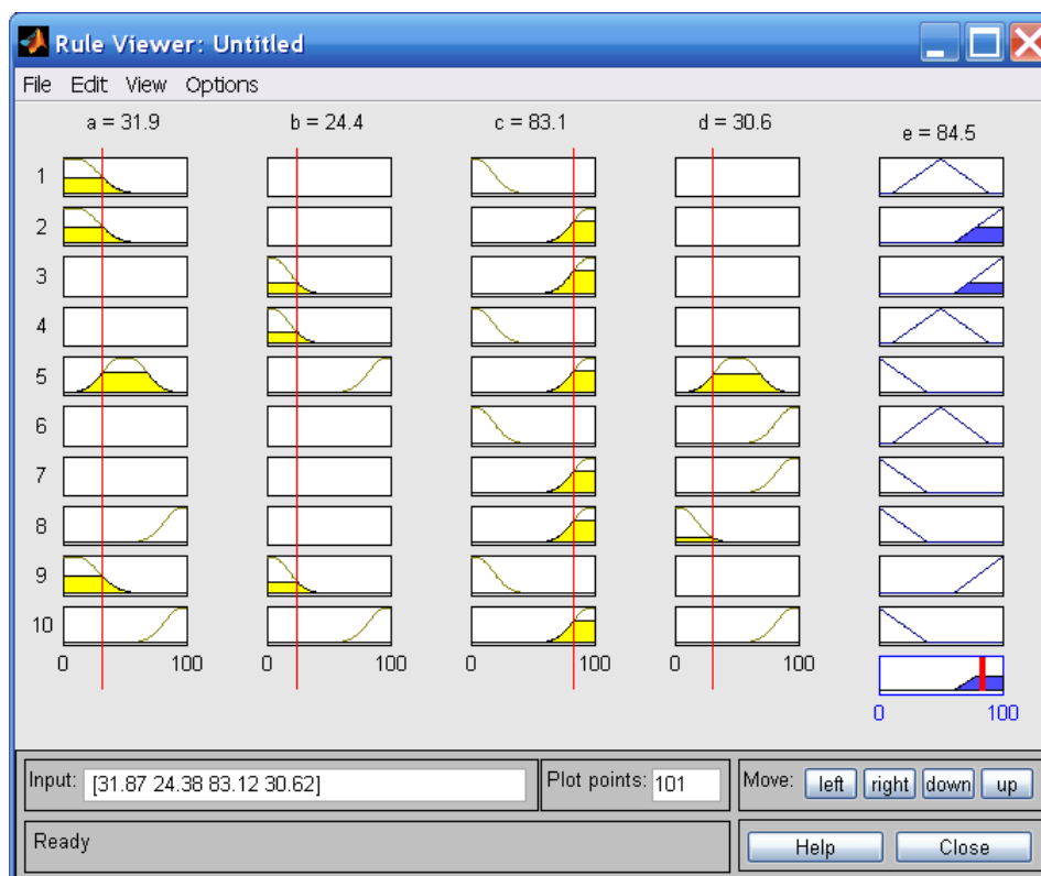
Рисунок 8 – Окно редактора вывода (входы 32, 24, 83, 31, результат – прогнозируемые затраты на ремонт - 85)
