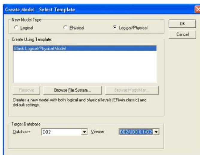
Рисунок 1.Создание новой модели
