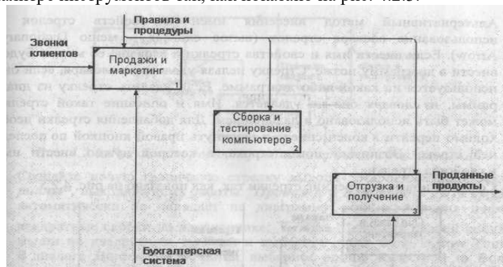
Рис. 4.2.3. Священные граничные стрелки на диаграмме АО
