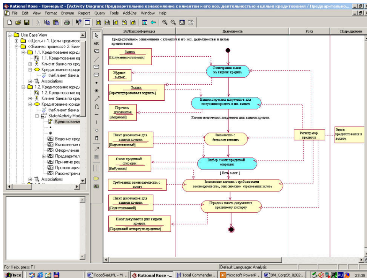
Рис. Пример изображения диаграммы с детальным описанием шага Предварительное ознакомление с клиентом и его хоз. деятельностью и целью кредитования в Rational Rose
