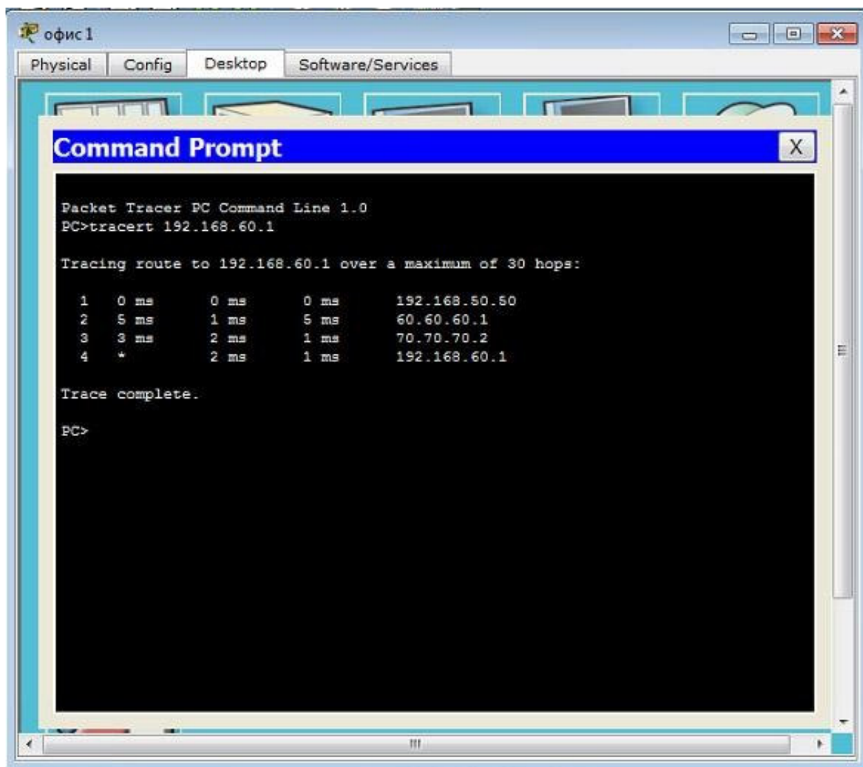
Рис. 6.4 – Трассировка
