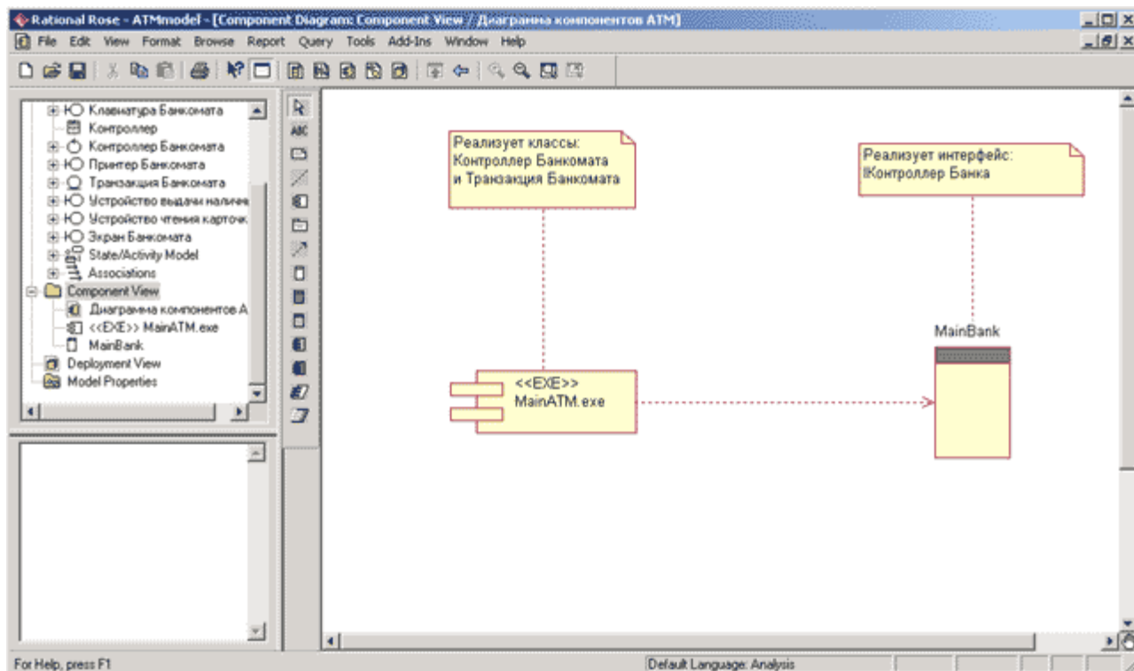
Рис. 12.4. Диаграмма компонентов после добавления отношения зависимости между компонентами MainATM.exe и MainBank
