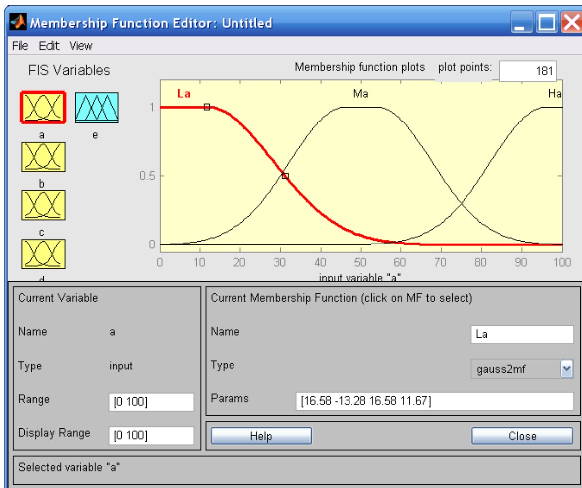
Рисунок 5 – Окно редактора функций принадлежности
