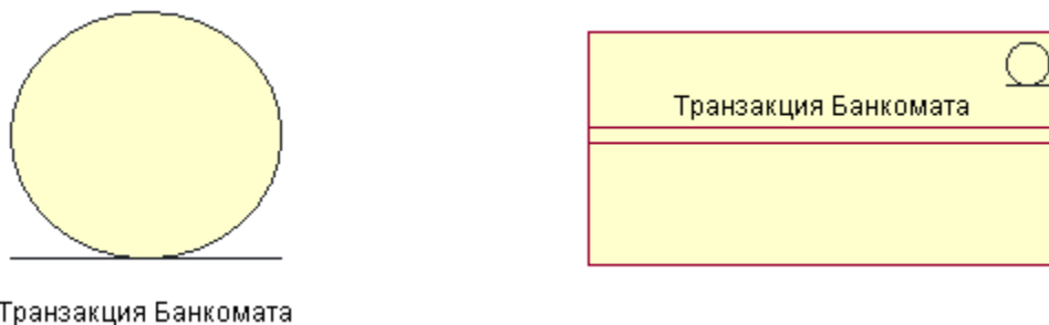
Рис. 4.5. Графические способы изображения стереотипа <<entity>> для класса Транзакция Банкомата
