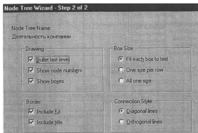
Рис. 4.4.2. Второй диалог гuida Node Tree Wizard
