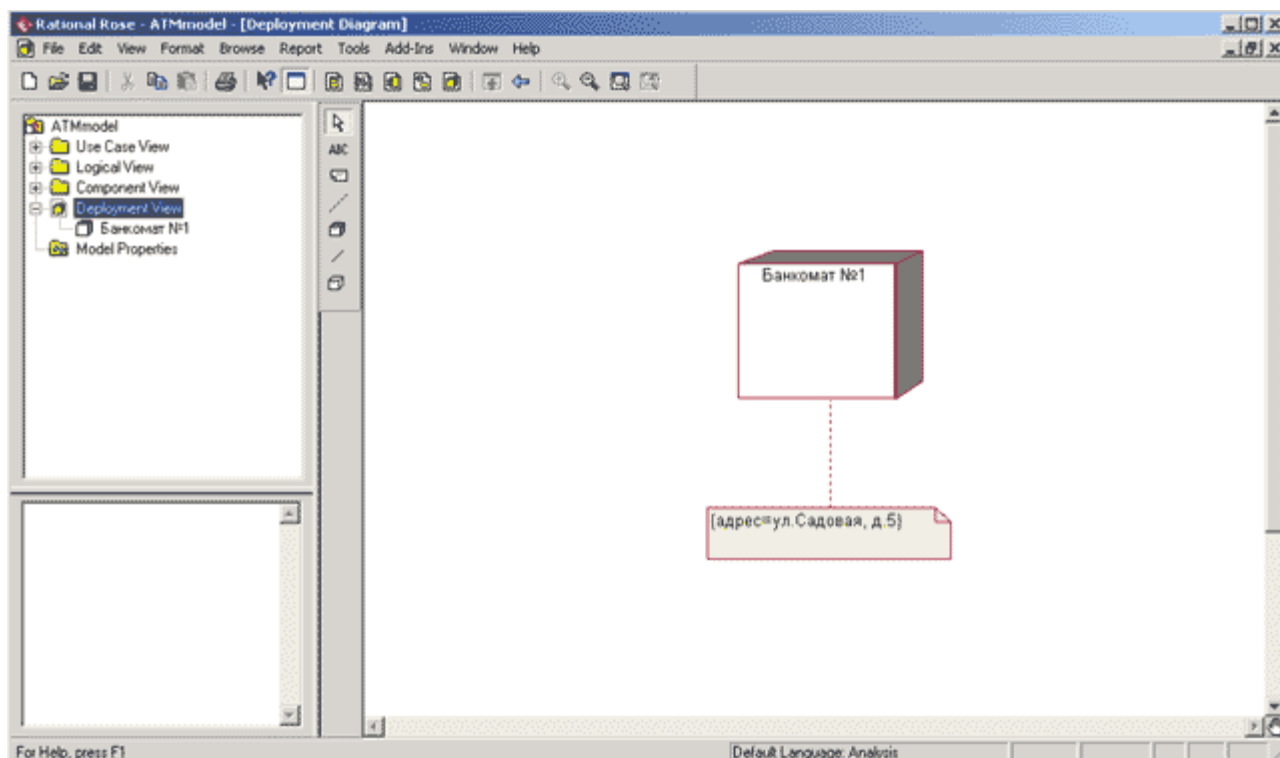
Рис. 13.1. Диаграмма развертывания после добавления узла Банкомат № 1
