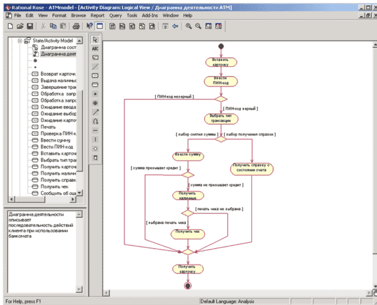
Рис. 10.5. Окончательный вид диаграммы деятельности для модели банкомата
