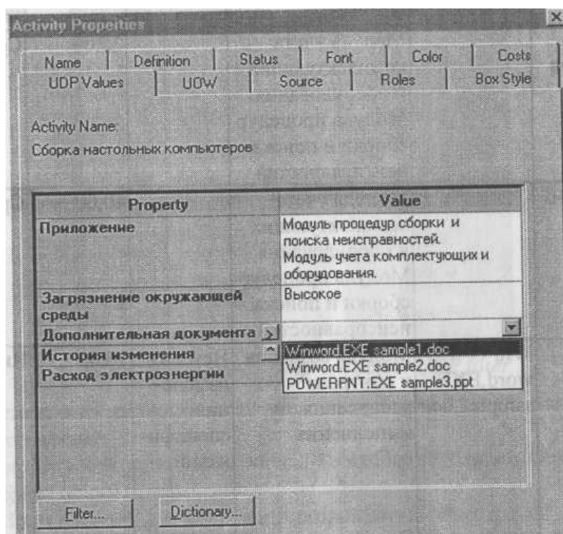
Рис. 4.10.3. Вкладка UDP Values диалога Activity Properties
