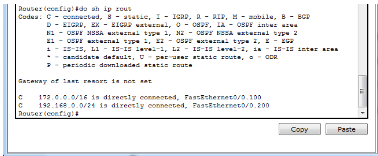
Рис. 8.2 – Таблица маршрутизации
