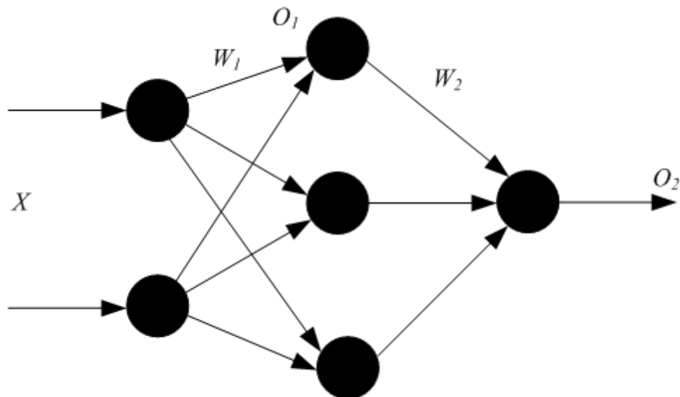
Рис. 5. Многослойный персептрон
