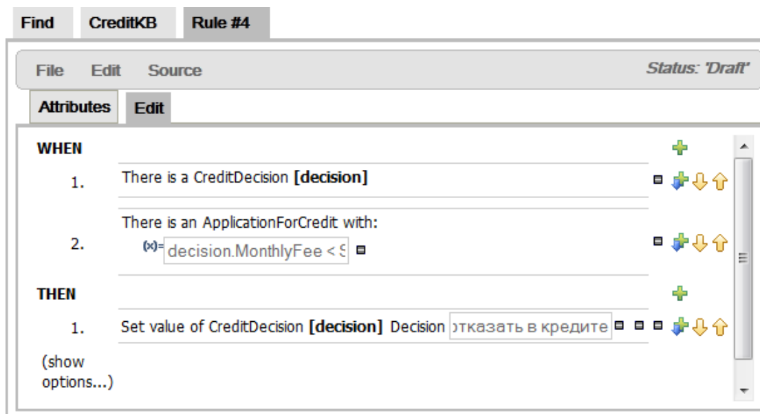
Рисунок 27 - Правило Rule #4
