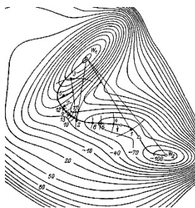
Рис. 1. Поверхность потенциальной энергии системы
