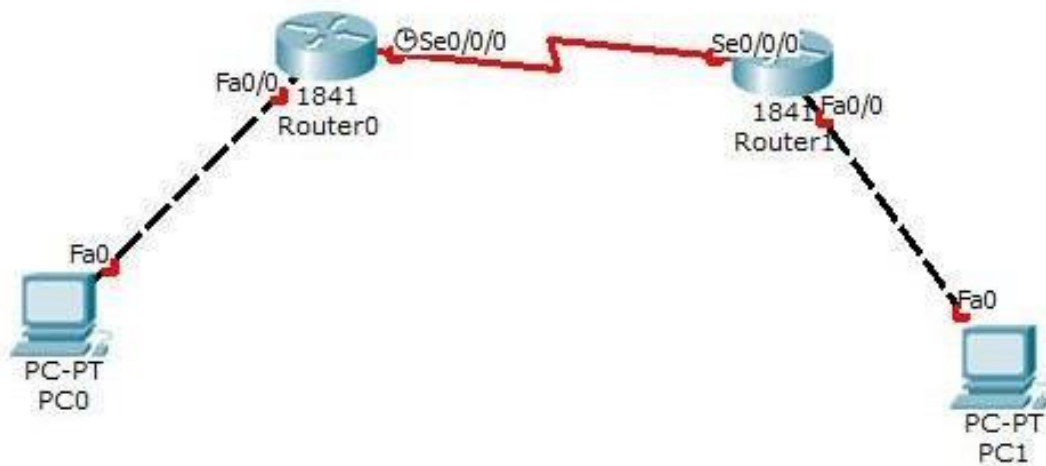
Рис. 5.1 – Топология сети
