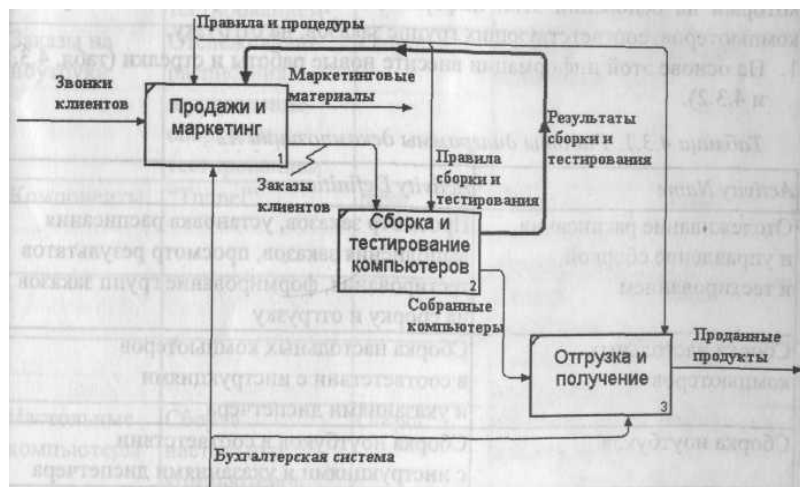
Рис. 4.2.7. Результат выполнения упражнения 2 - диаграмма АО
