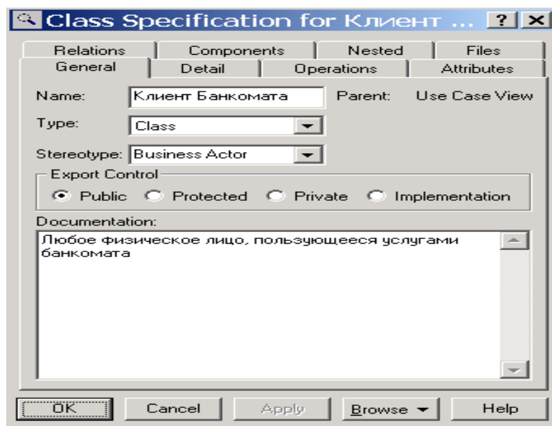
Рис. 3.5. Диалоговое окно спецификации свойств после изменения стереотипа и добавления текста документации для актера Клиент Банкомата
