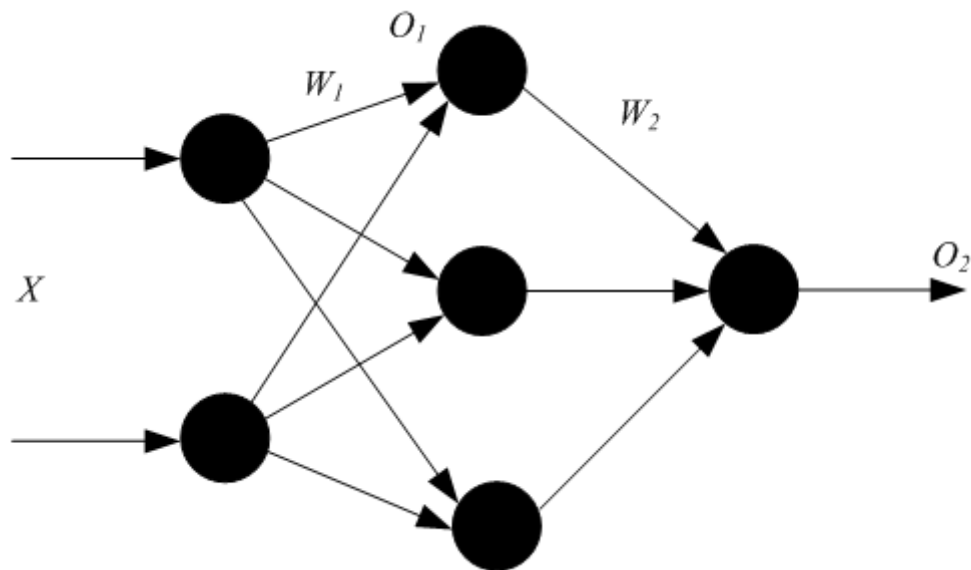
Рис. 5. Многослойный персептрон
