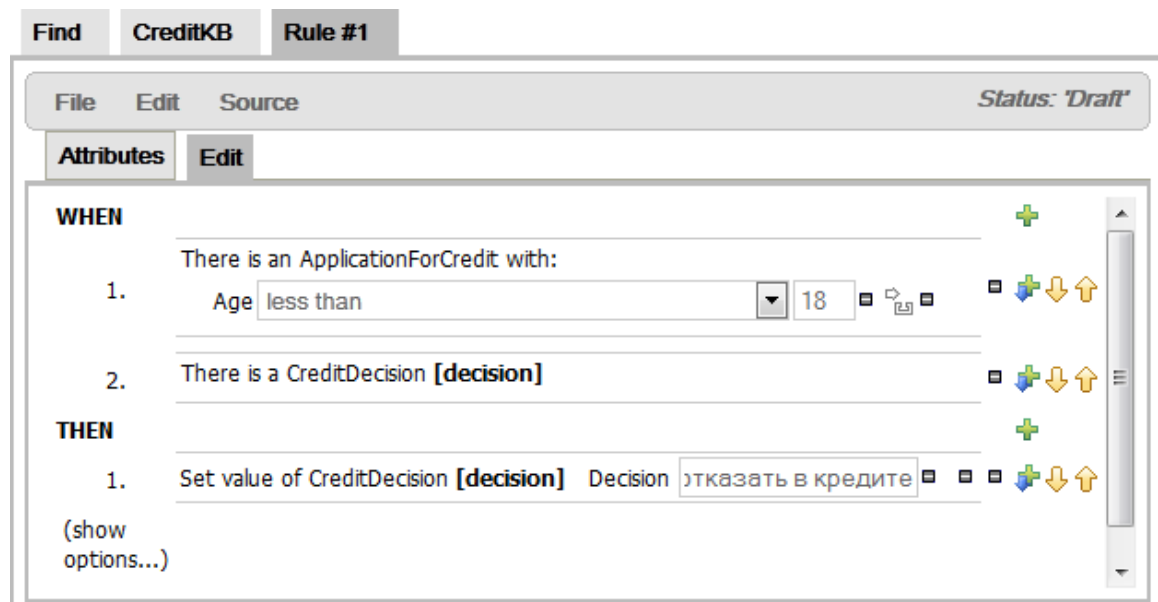
Рисунок 20 - Законченное правило
