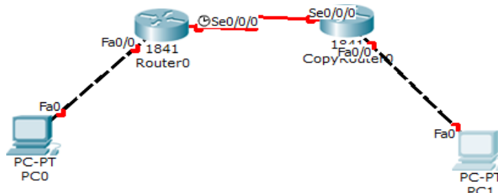
Рис 7.1 – Топология EIGRP
