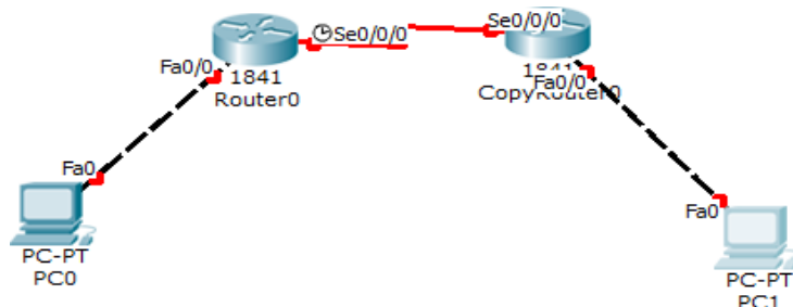
Рис 7.1 – Топология EIGRP
