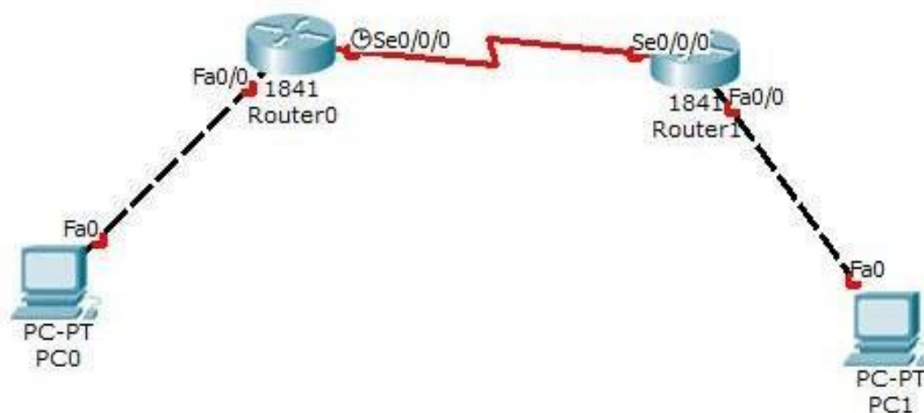
Рис. 5.1 – Топология сети
