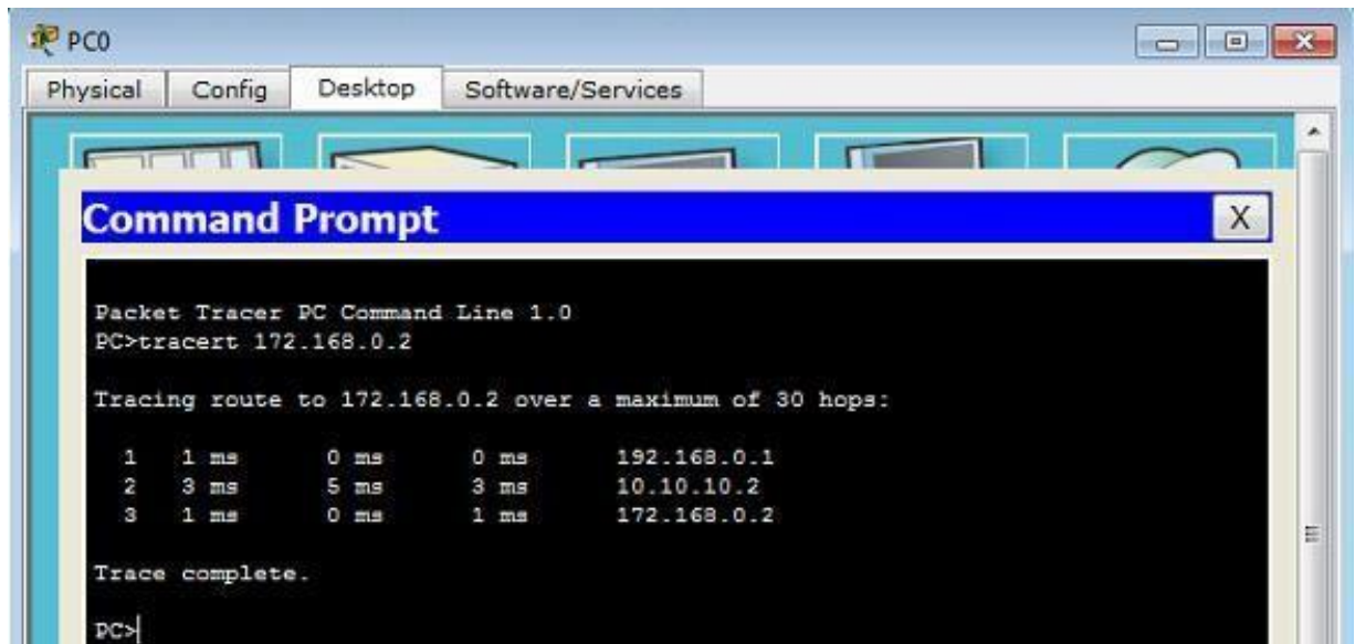
Рис. 7.3 – Трассировка
