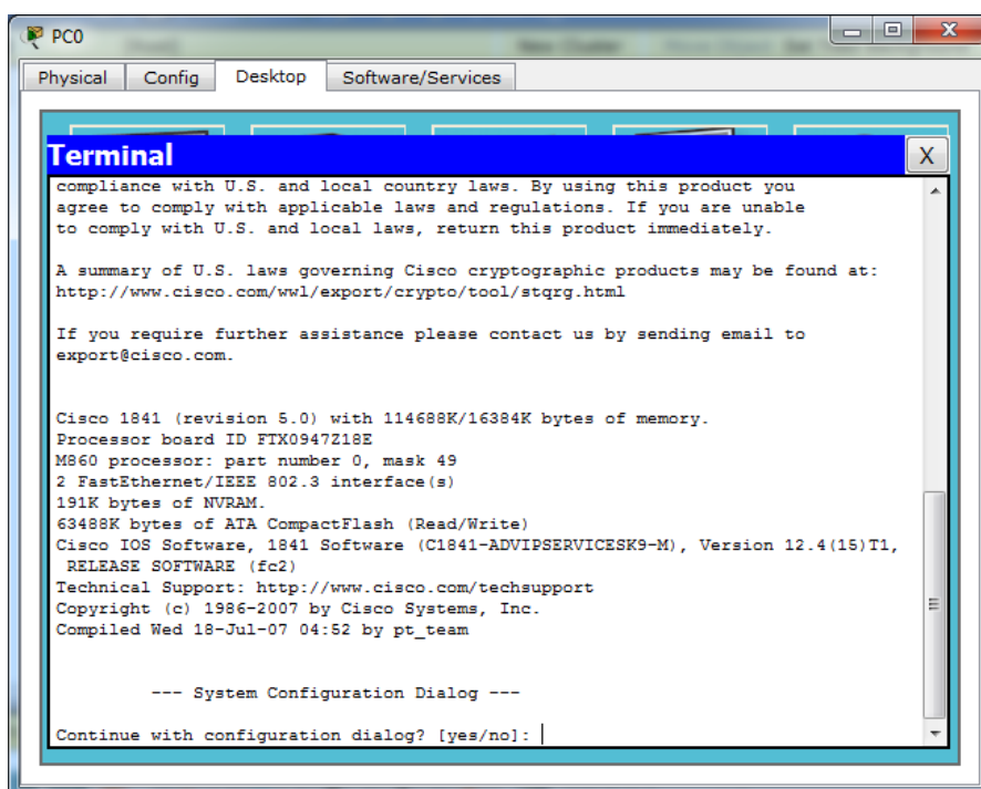
Рис. 3.3 – Командная строка CLI
