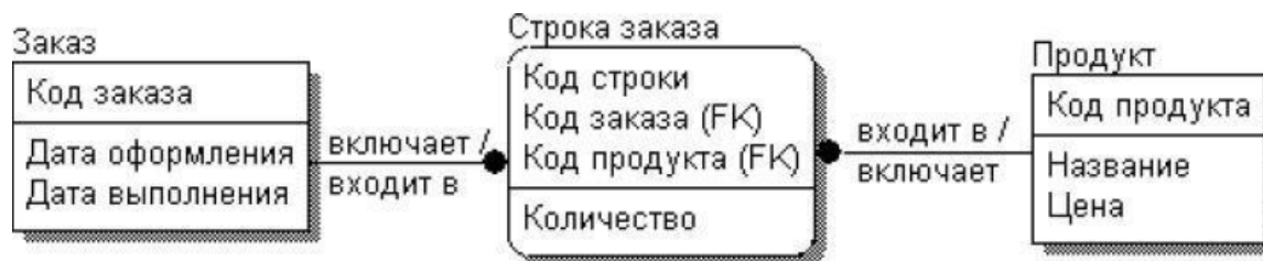
Рисунок 8. Автоматически созданная физическая схема БД
