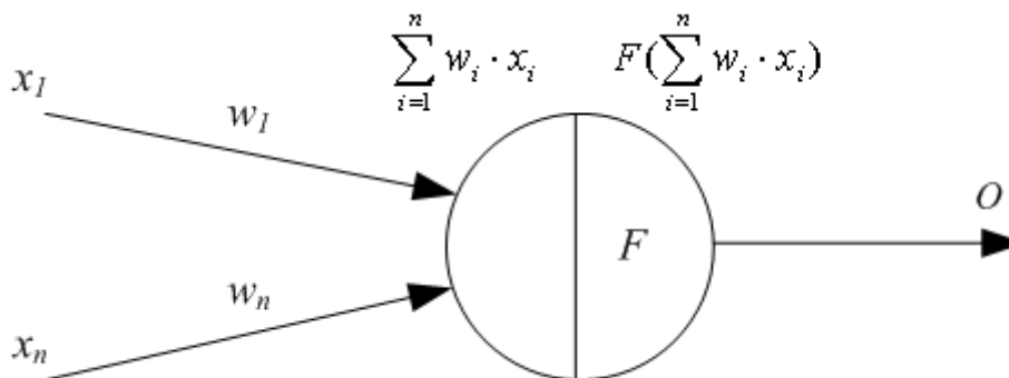
Рис. 1. Искусственный нейрон
