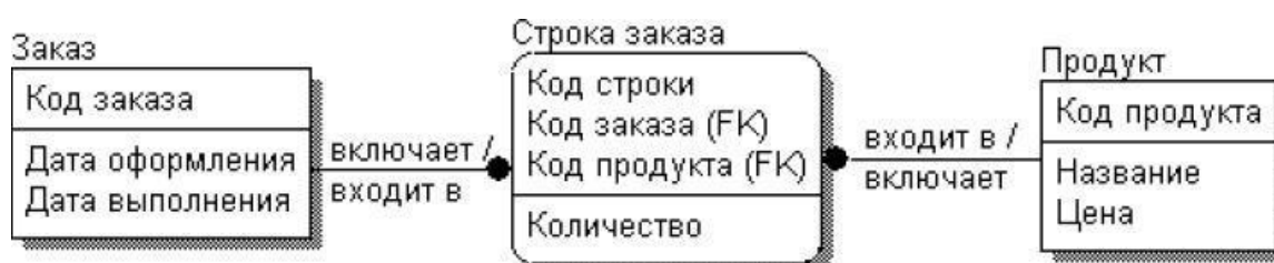
Рисунок 7.Пример логической схемы БД
