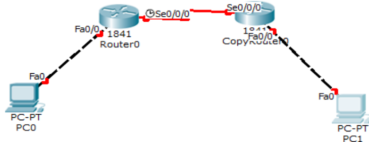
Рис 7.1 – Топология EIGRP
