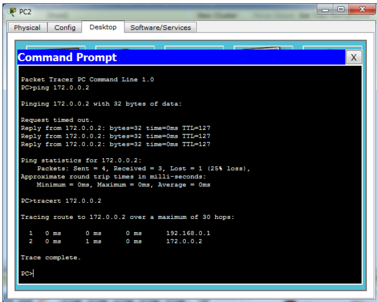
Рис. 8.3 – Трассировка
