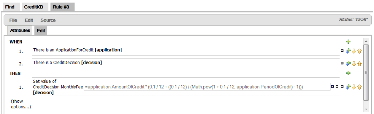
Рисунок 25- Правило Rule #3
