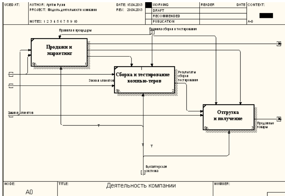
Рисунок 3. Декомпозиции А-0
