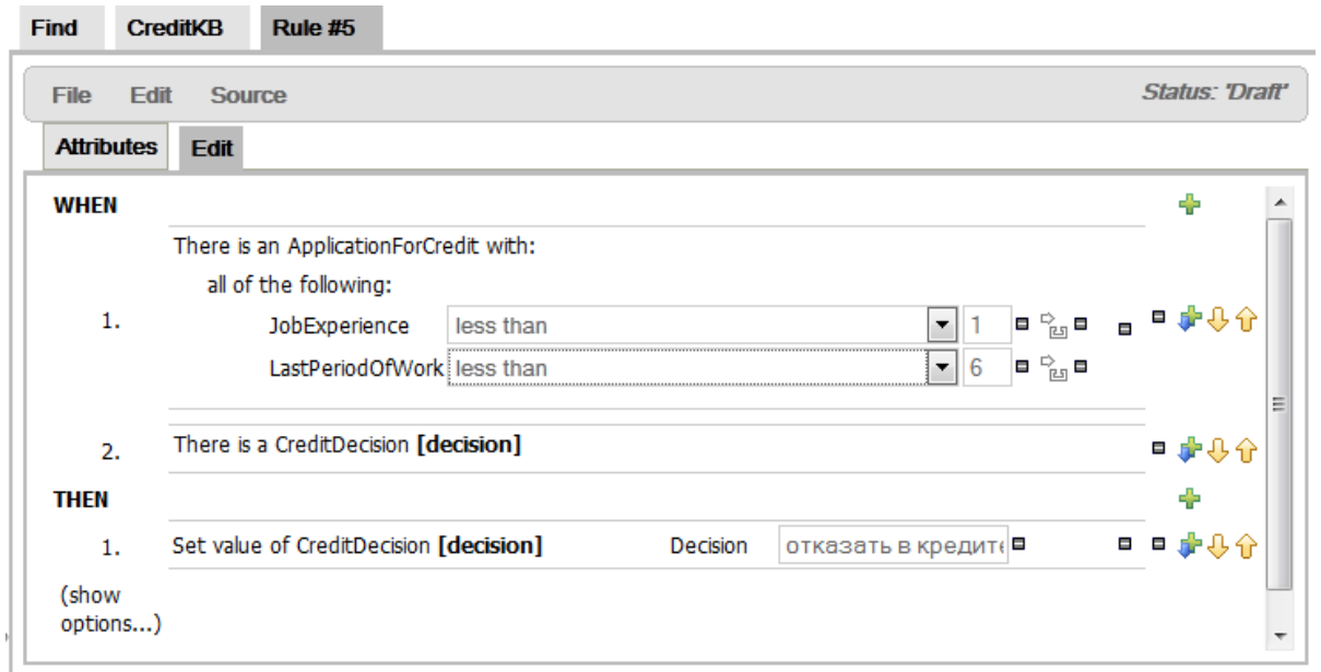
Рисунок 30 - Правило Rule #5
