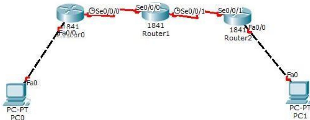
Рис. 4.1 – Топология сети
