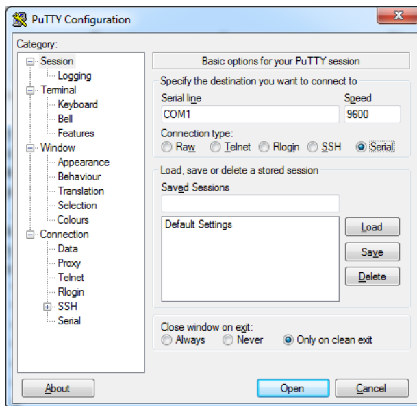
Рис. 3.1 – Окно подключения программы Putty
