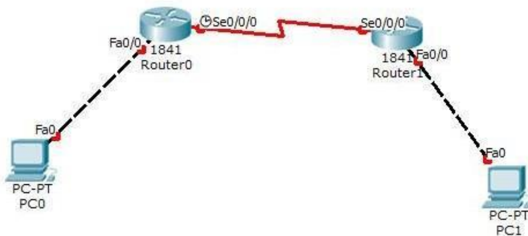
Рис. 5.1 – Топология сети
