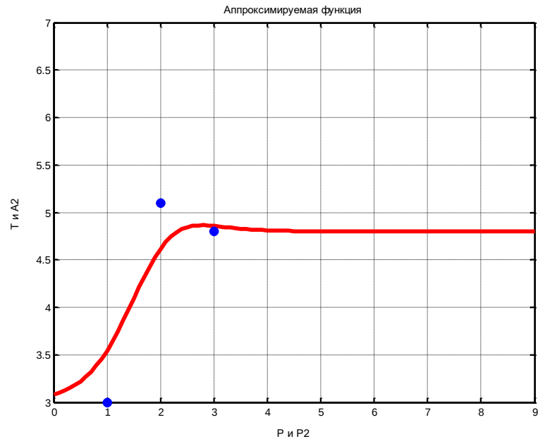
Рис. 9. Аппроксимация точек с помощью нейронной сети регрессии
