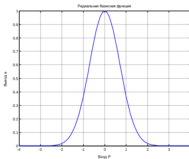
Рис. 10. Радиальная базисная функция
