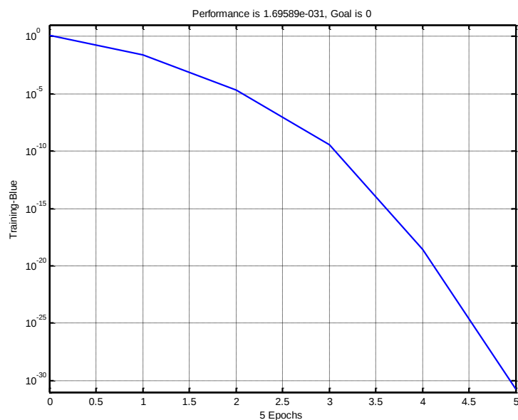
Рис. 6. График обучения двухслойного персептрона
