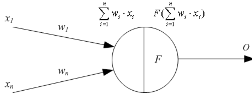
Рис. 1. Искусственный нейрон
