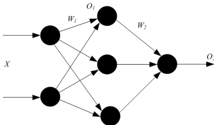
Рис. 5. Многослойный персептрон
