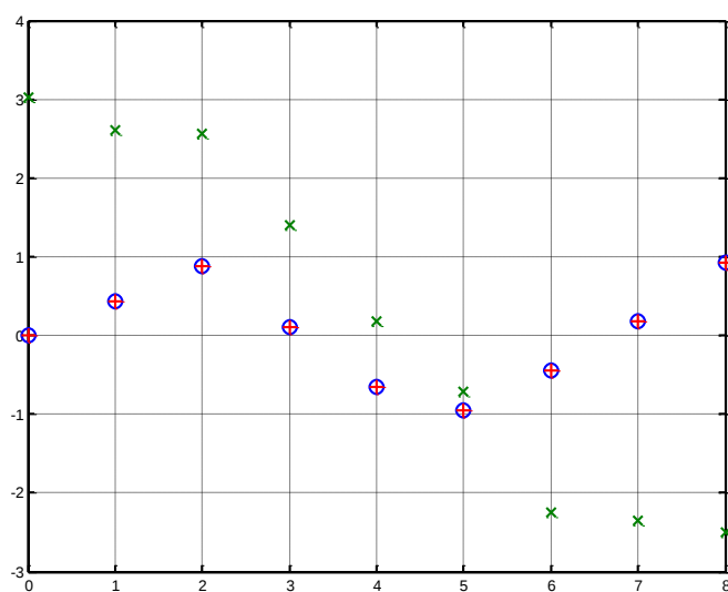
Рис. 7. Результат аппроксимации векторов двухслойным персептроном
