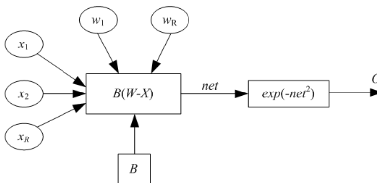
Рис. 8. Радиальный базисный нейрон
