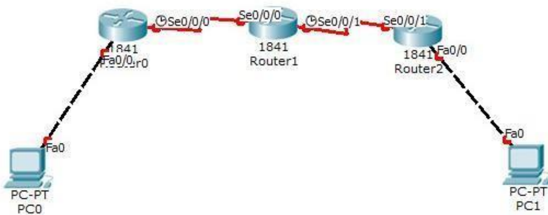
Рис. 4.1 – Топология сети
