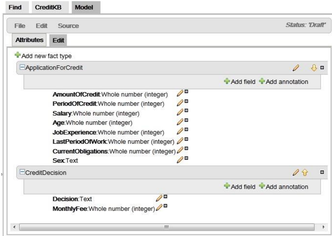
Рисунок 11 - Вкладка модели базы знаний
