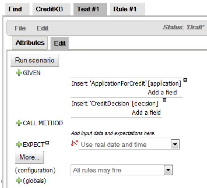
Рисунок 33 - Тест Test #1 и входные факты
