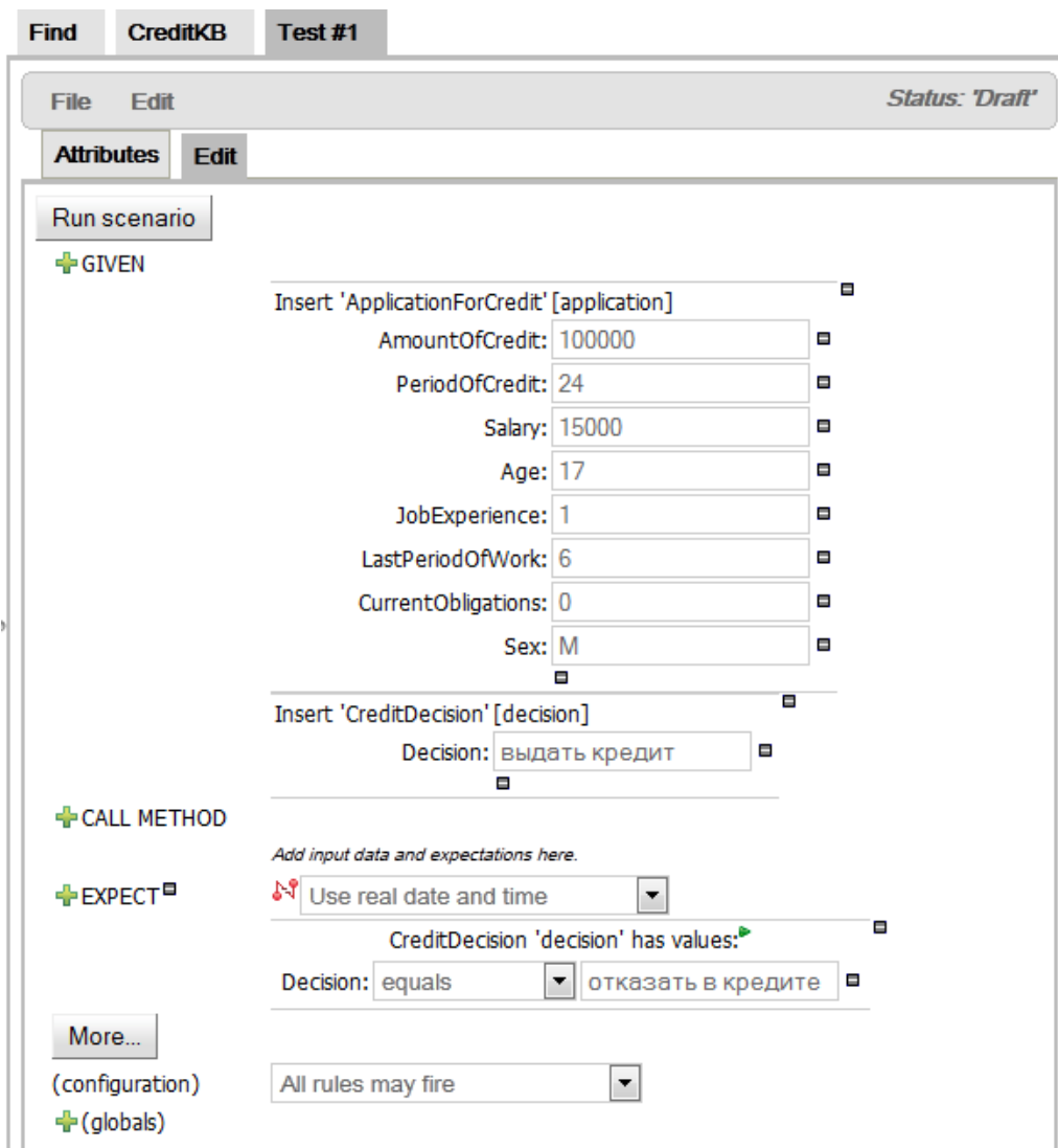
Рисунок 35 - Тестовый сценарий Test #1
