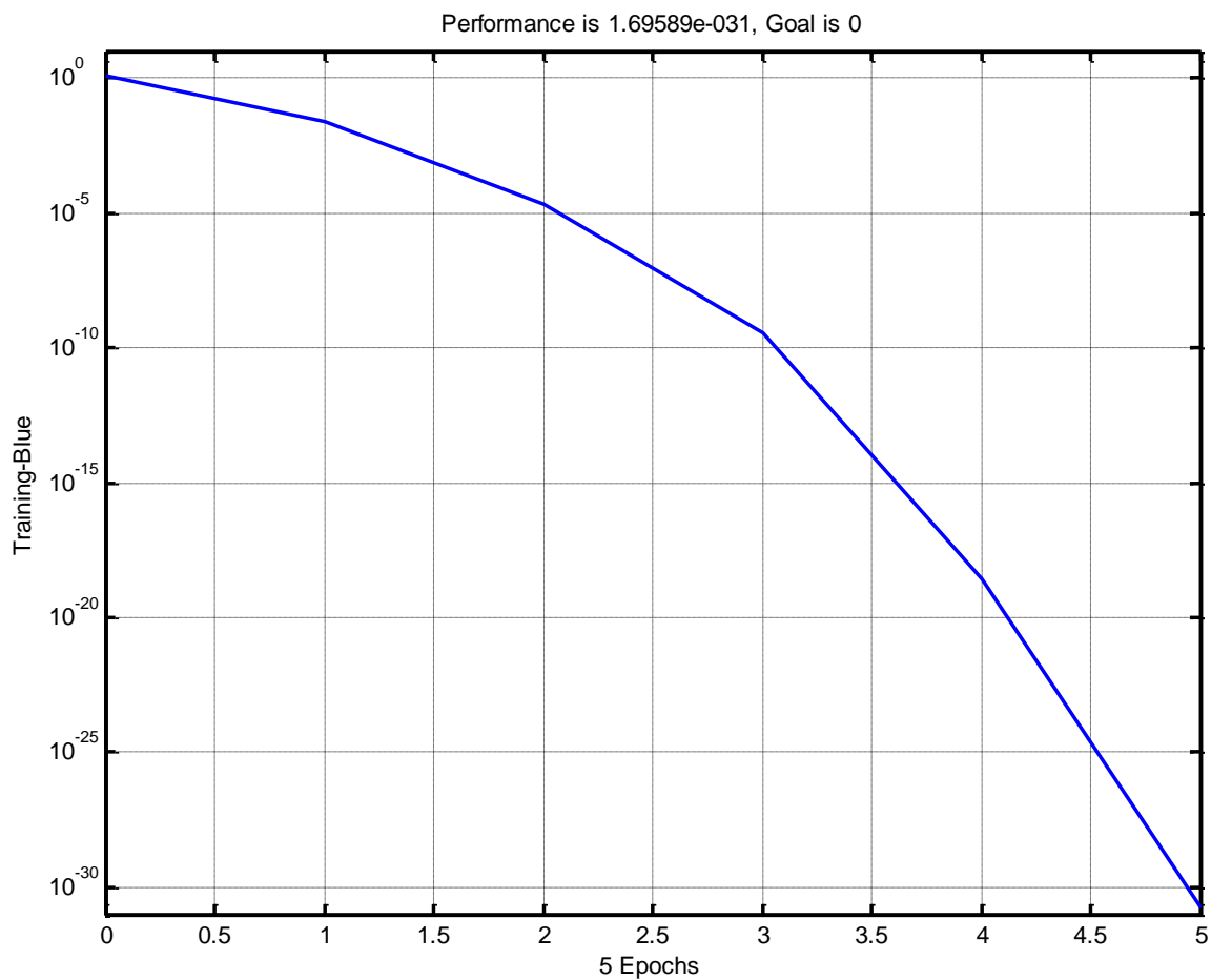
Рис. 6. График обучения двухслойного перцептрона
