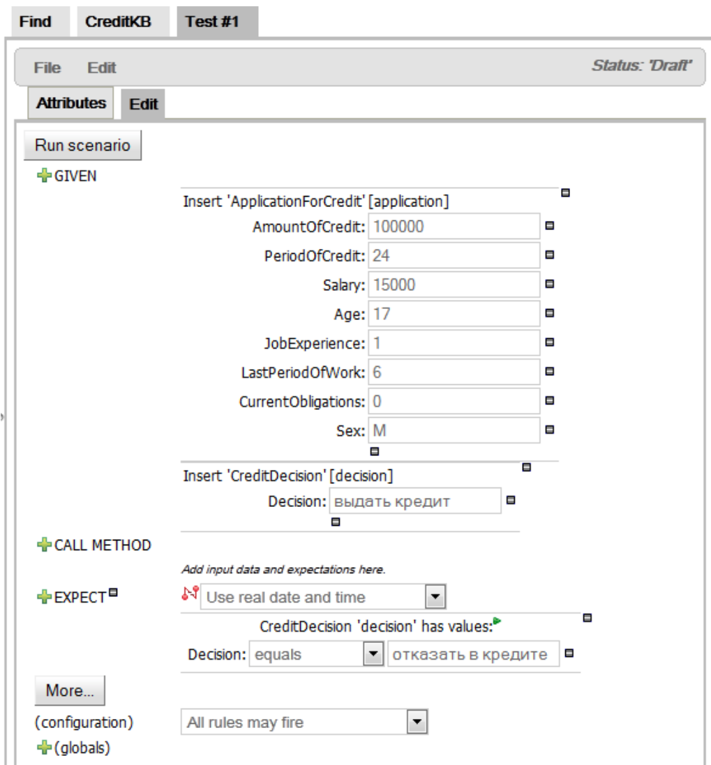
Рисунок 35 - Тестовый сценарий Test #1
