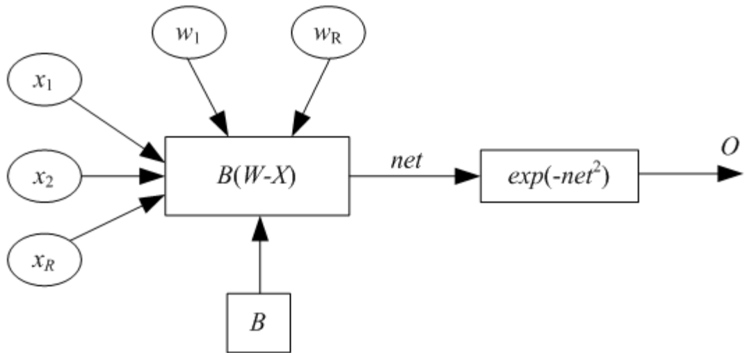
Рис. 8. Радиальный базисный нейрон
